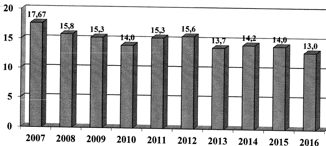
Lyginamosios elektros energijos sąnaudos šilumos gamyboje, kWh e /MWh
